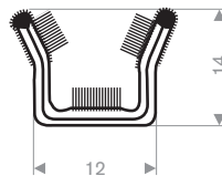
219.01.022 EPDM + textiel
